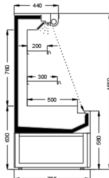
Marbella 56.A1 H:1550
