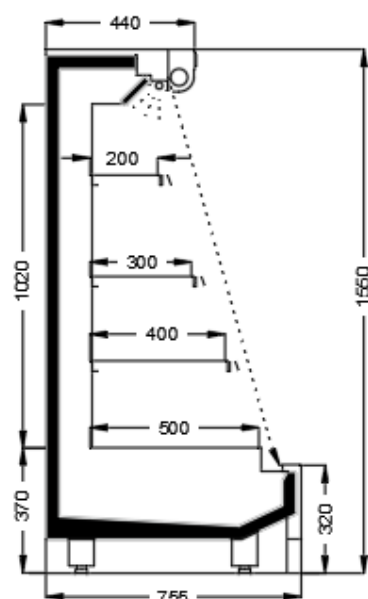
Marbella 53.A1 H:1550
