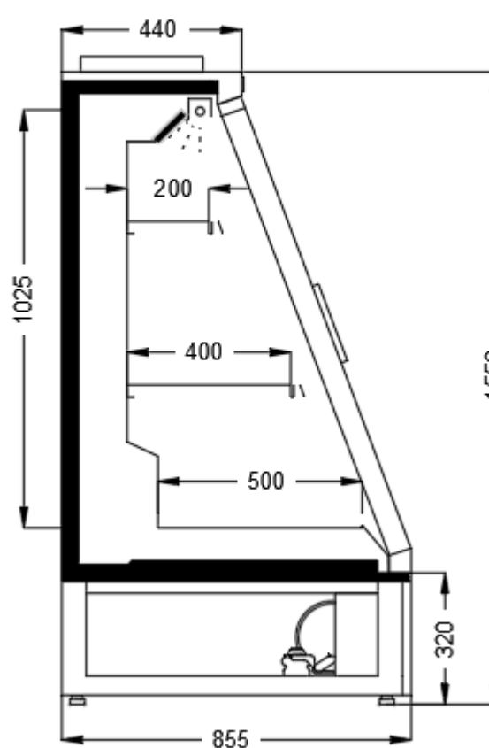
Macon 53.A3.SGD H:1550
