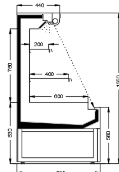
Marbella 66.A1 H:1550
