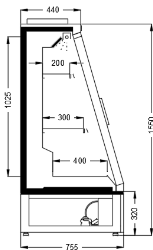
Macon 43.A3.SGD H:1550
