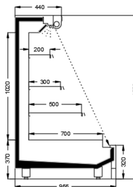
Marbella 73.A1 H:1550
