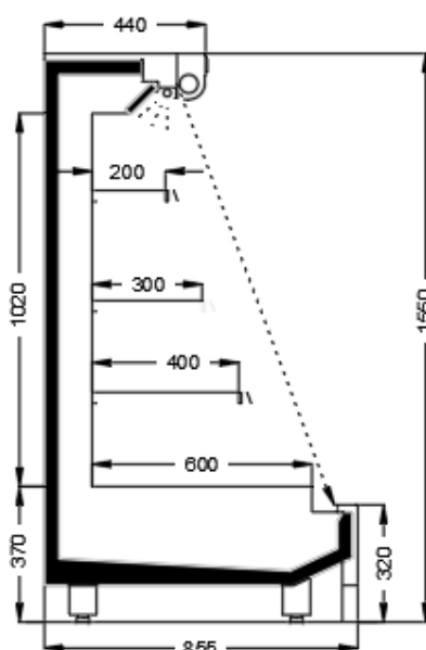
Marbella 63.A1 H:1550
