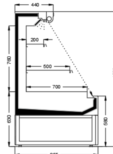
Marbella 76.A1 H:1550
